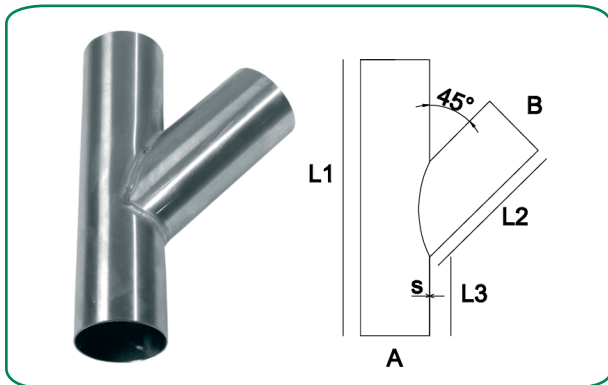
STBP grenrør elektrogalvanisert , avgrening 45 gr.
