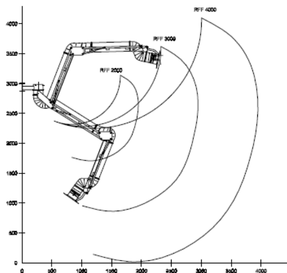
Rækkevidde RFF-A 2000 - 4000 (ø160mm):
