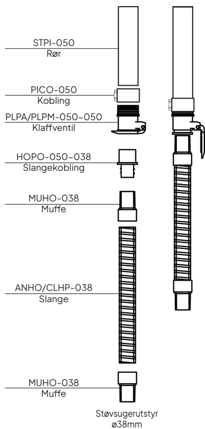
PLPA / PLPM Eksempel: \varnothing 50 rør, \varnothing 38 slange
