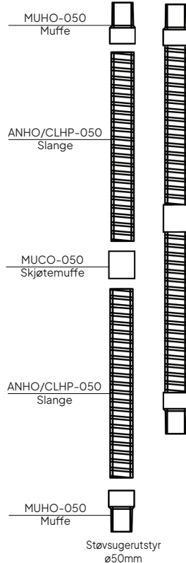
Slangeforlenger Eksempel: \varnothing 50 slange
