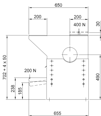
Støvsuffe Enkel tilgang til støvsuffe for tømning.
