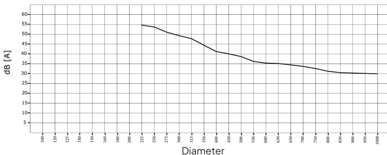
GASI-B L=1000 mm lyddempingstabell
