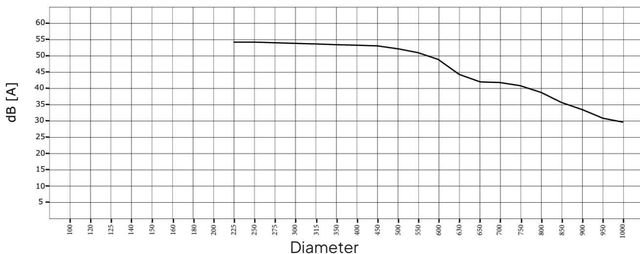
GASI L=2000 mm lyddempingstabell
