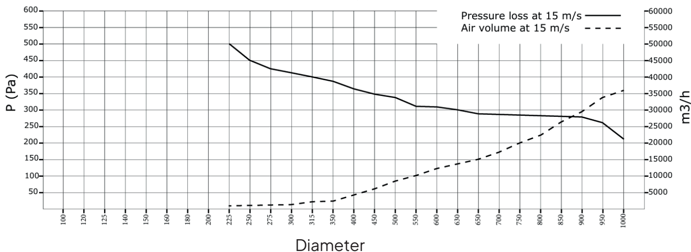
GASI L=2000 mm trykkfallstabell
