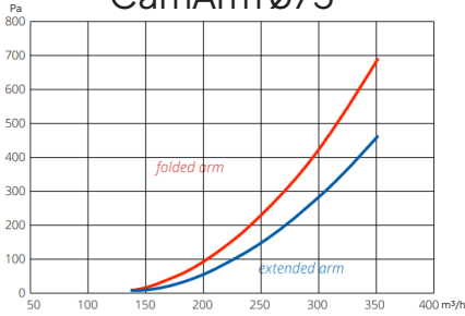
CamArm \varnothing 75
