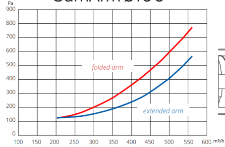
CamArm \varnothing 100
