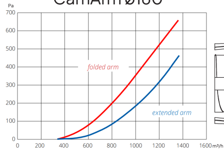
CamArm \varnothing 160
