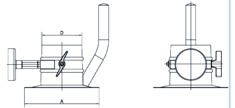
ST-M Sugetrakt med magnet og spjeld Type A D ST-MS-100 ø188 ø100 ST-MS-125 ø230 ø125 ST-MS-160 ø300 ø160
