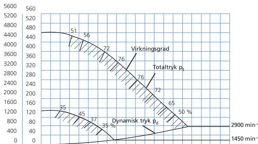
Virkningsgrad og tryk
