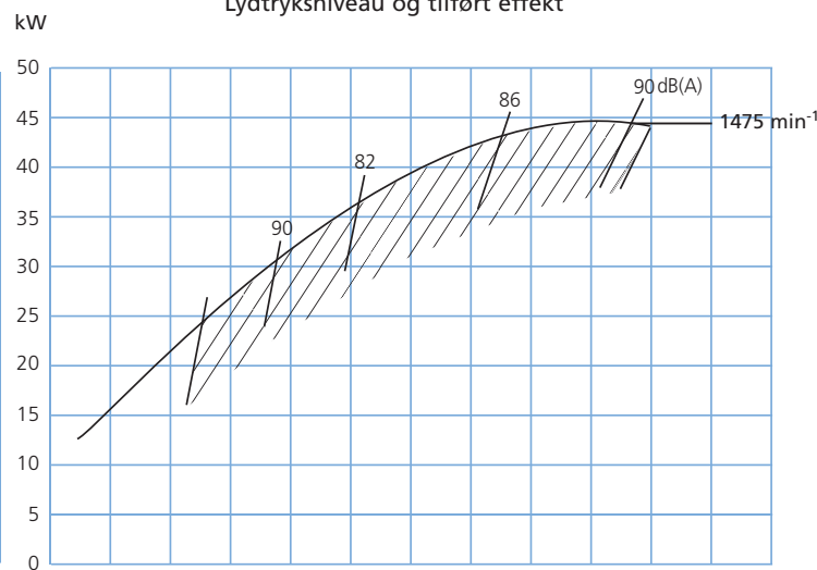
Lydtryksniveau og tilført effekt
