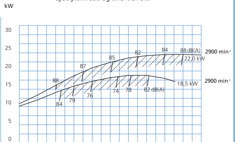
Lydtryksniveau og tilført effekt
