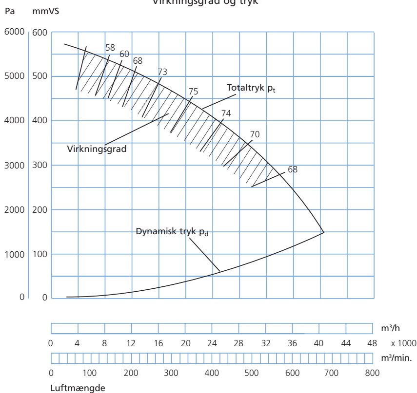
Virkningsgrad og tryk
