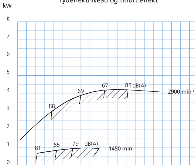
Lydeffektniveau og tilført effekt
