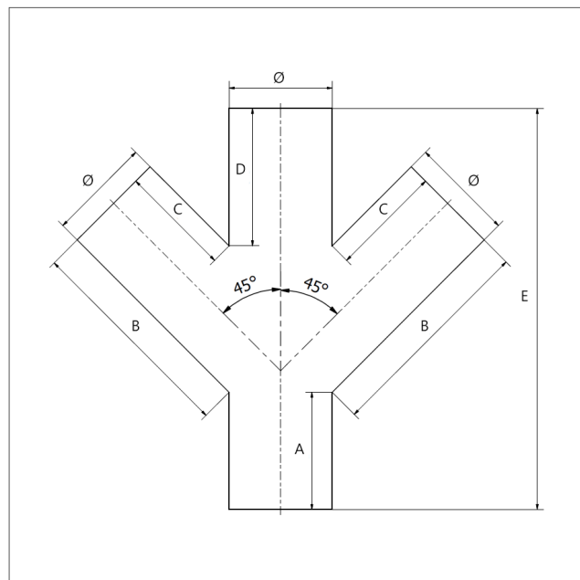
STBD - dubbelt grenrør, ritning. För mått - se tabell.
