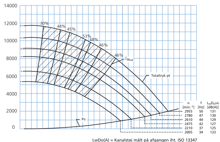
P_t [Pa] Total virkningsgrad og tryk
