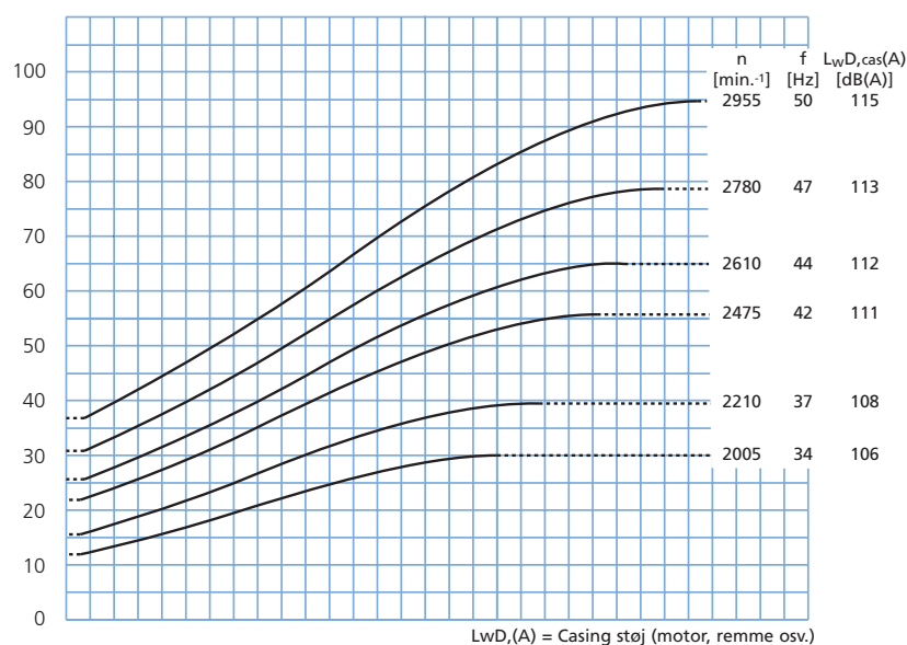
P_t [Pa] Total virkningsgrad og tryk
