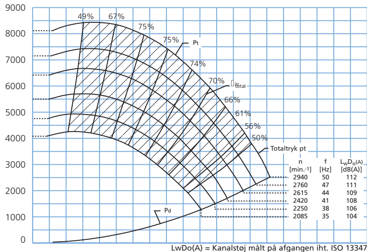
P t [Pa] Total virkningsgrad og tryk
