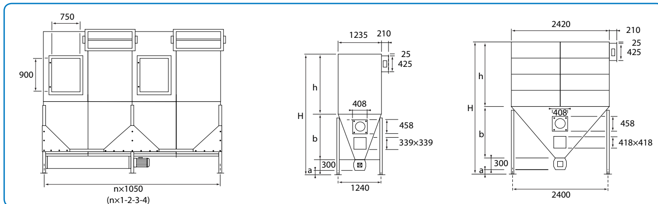
Tegningen herover viser enkelt- og dobbeltfilter. Målespesifikationer er angivet i skemaet nederst på siden.
